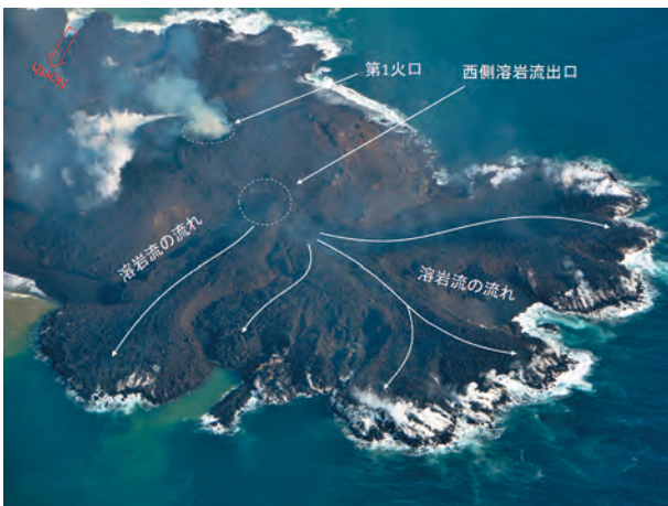
Photo 15. Number 1 crater and west side lava flow on December 13, 2013 (photo taken by Japan Coast Guard). 写真 15. 第1火口と西側溶岩流 (2013年12月13日 海上保安庁撮影).
